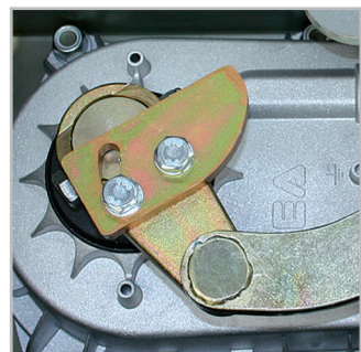
Stops mécaniques réglables dans les deux directions
